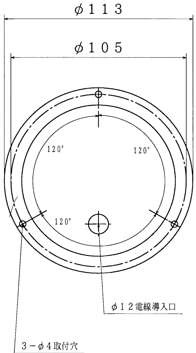
《取付け面寸法図》
